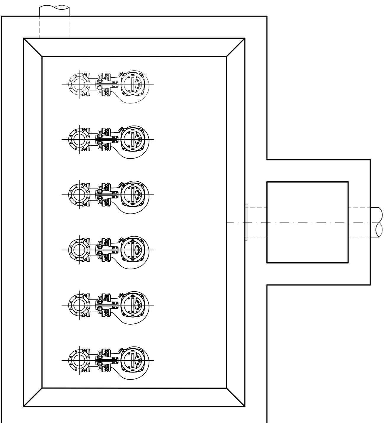
PLANTA DE FONDO. SALA DE BOMBAS
