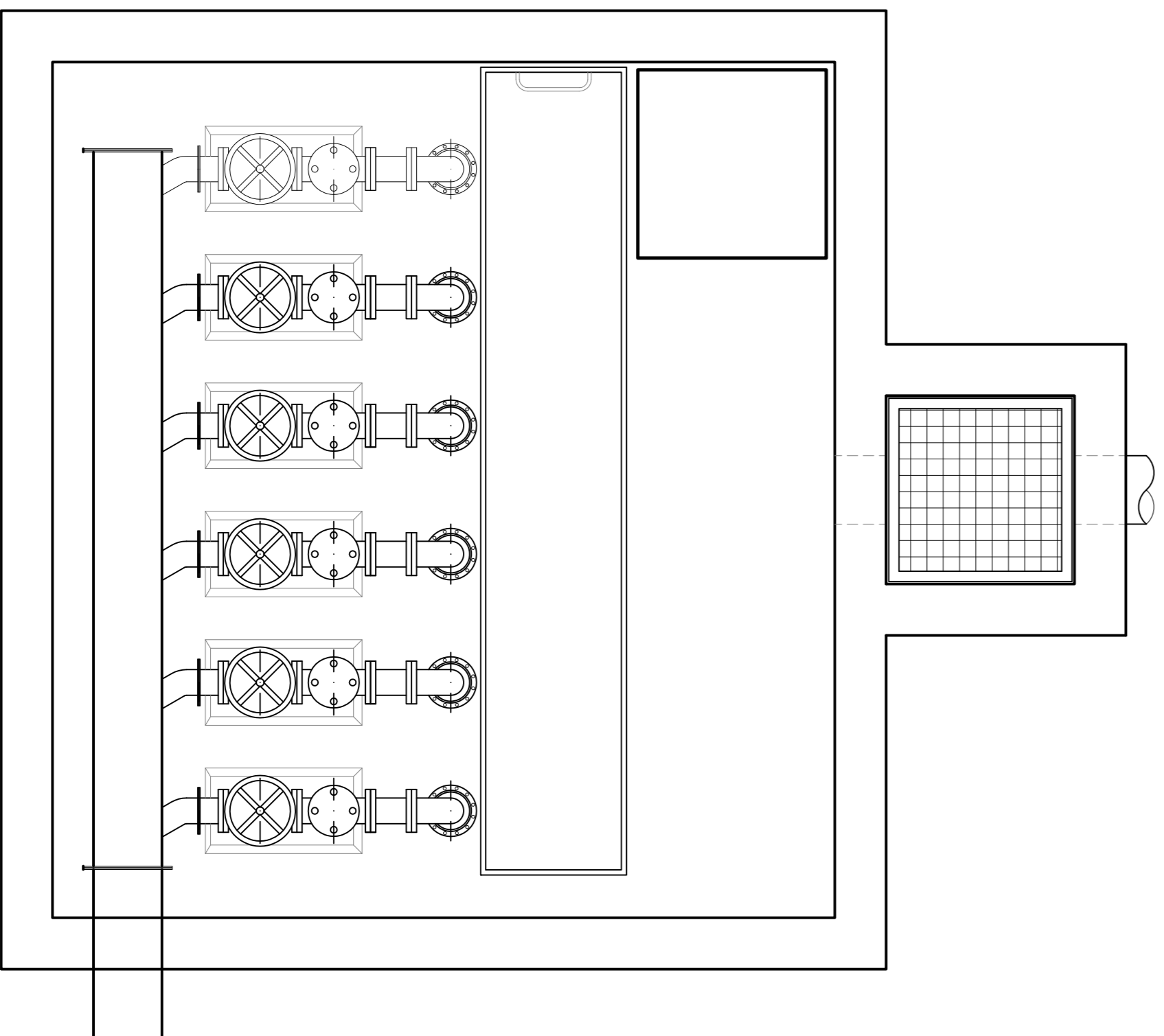
PLANTA INTERMEDIA. SALA DE VALVULAS
