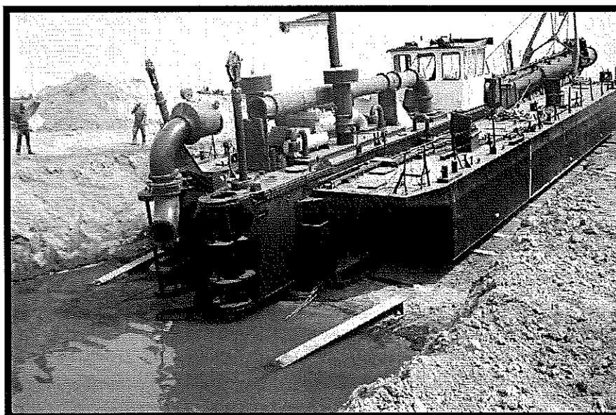
Botadura Draga en Río Salado
