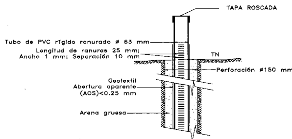
DETALLE DE LOS PIEZOMETROS
