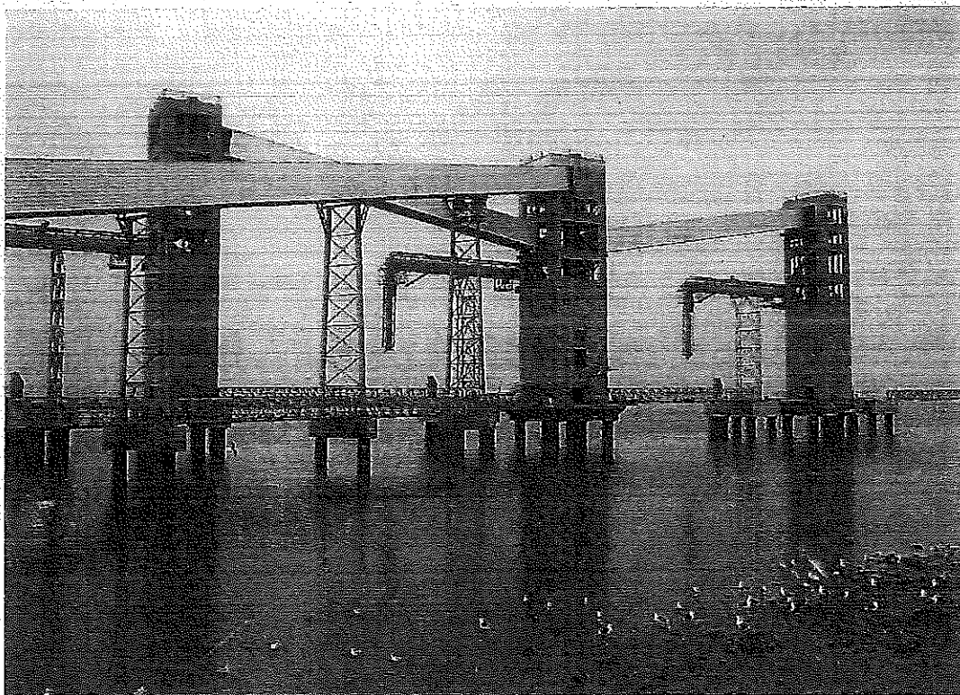
OBRA CIVIL MUELLE ALFRED C. TOEPFER Y SUS COMPLEMENTARIAS. ING. WHITE B. BLANCA, BUENOS AIRES ARGENTINA
