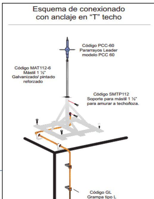
Esquema de instalación de pararrayos .Ver Plano IE-01
