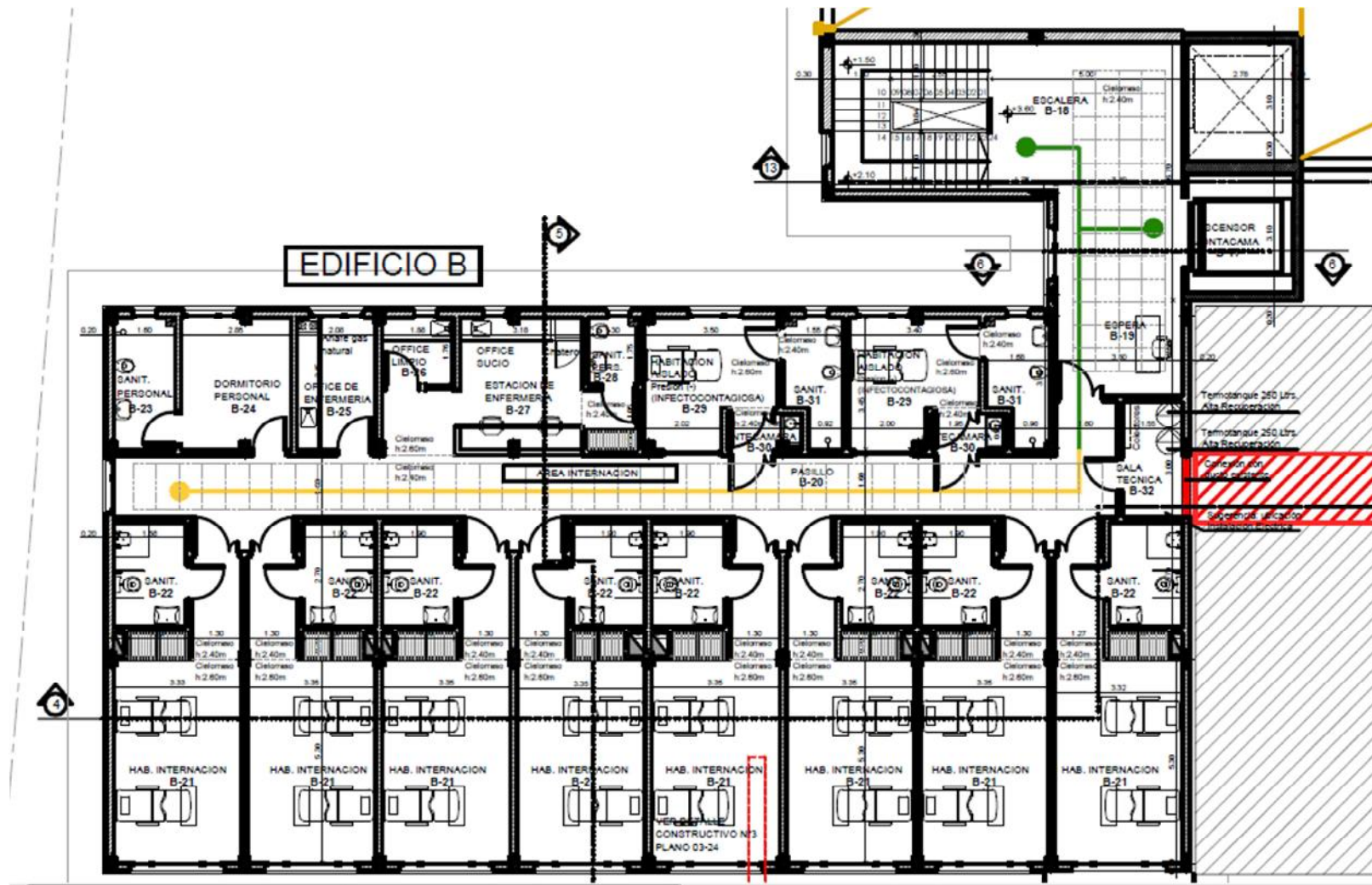
Figura N° 7: Primer piso del sector de internación.
