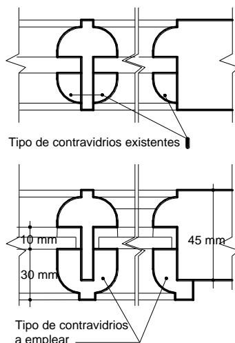
Figura 1: Reemplazo de Contravidrios para vidrios de seguridad
