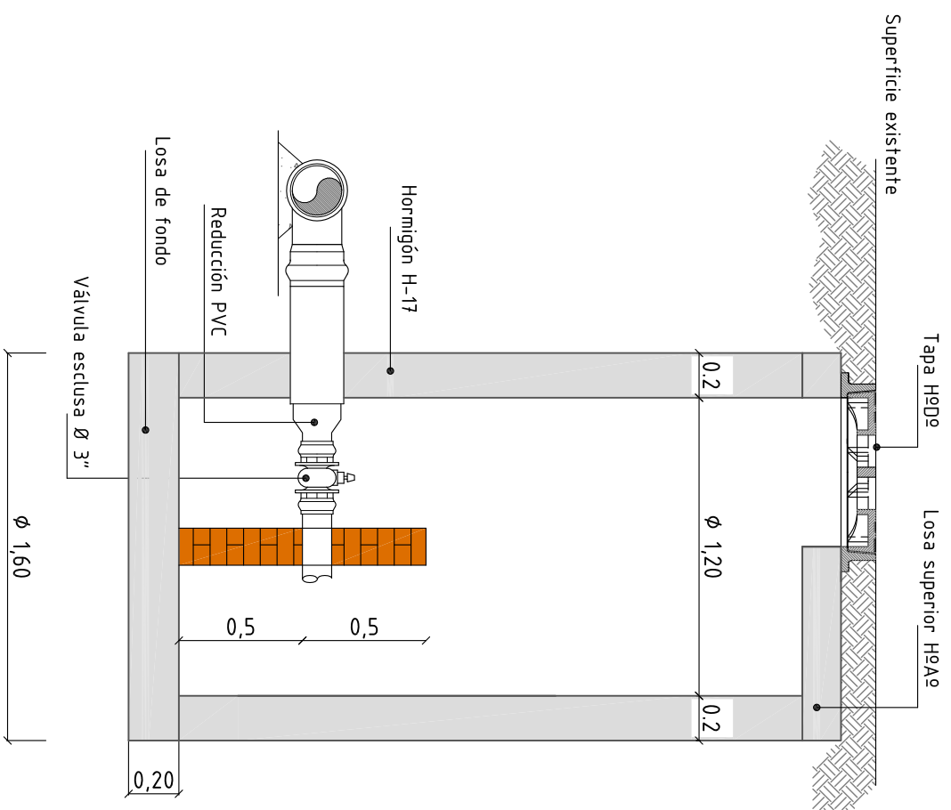
CORTE A-A
