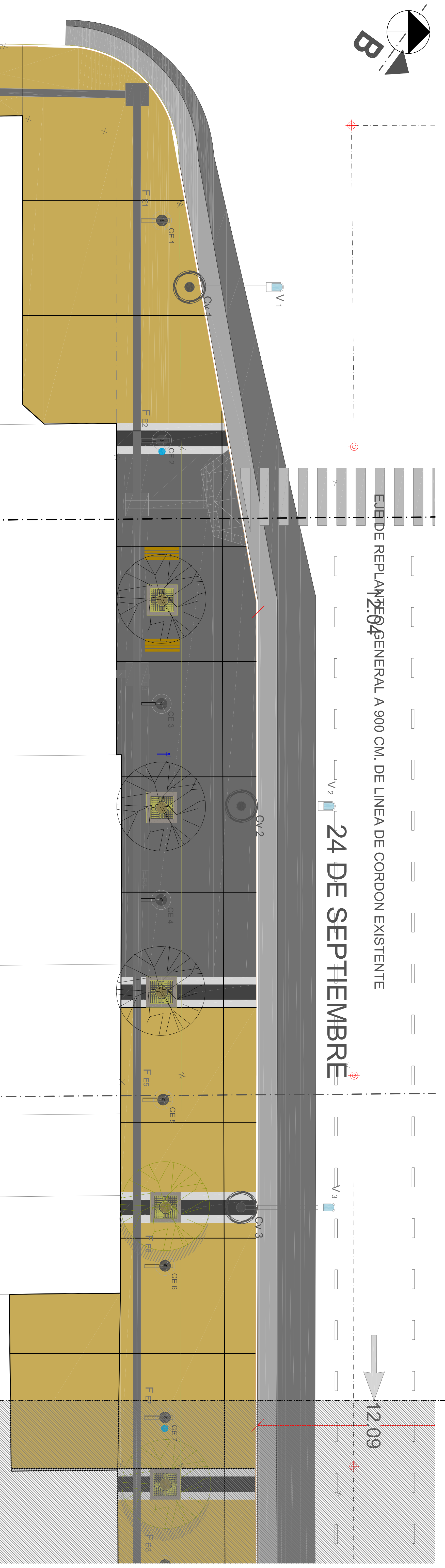
SECTOR OESTE | CALLE 24 DE SEPTIEMBRE | JUNTAS DE DILATACION | 1 : 100
