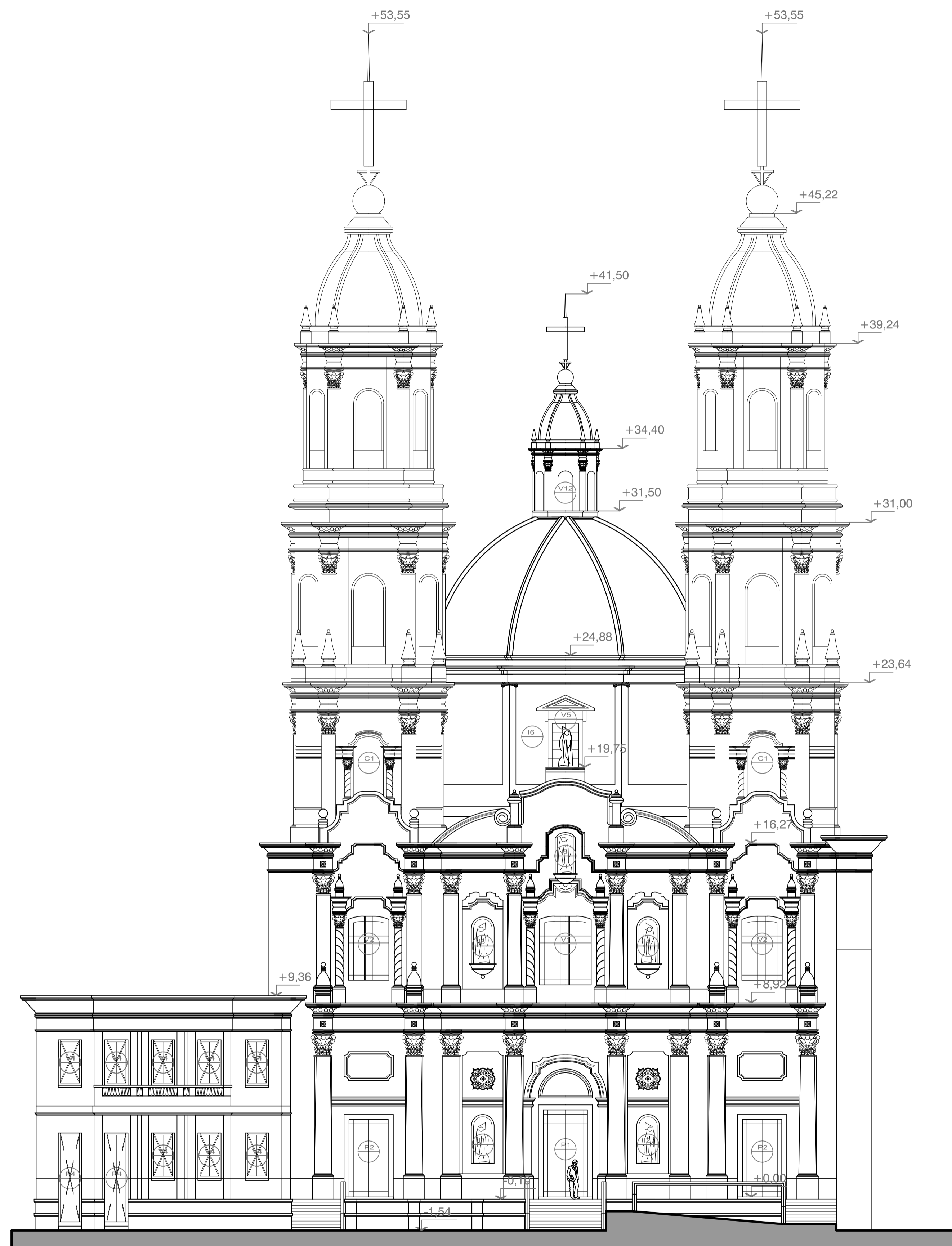
FACHADA SOBRE L.M ESC. 1:125
