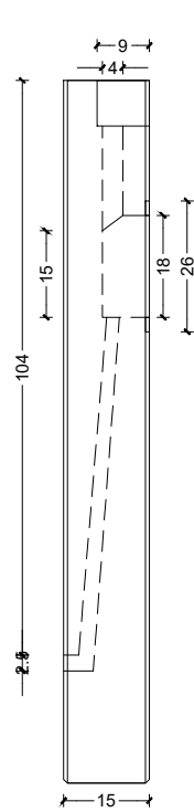
VISTA LATERAL
